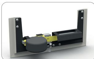
Měřicí přípravek na síť -pro profil R50 33 x 11 mm
