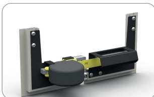
Měřicí přípravek na síť -pro profil LEM 12 x 11 mm
